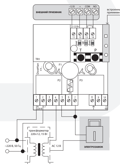
Рис. 3. Схема подключения электрозамка к DoorHan CV01
