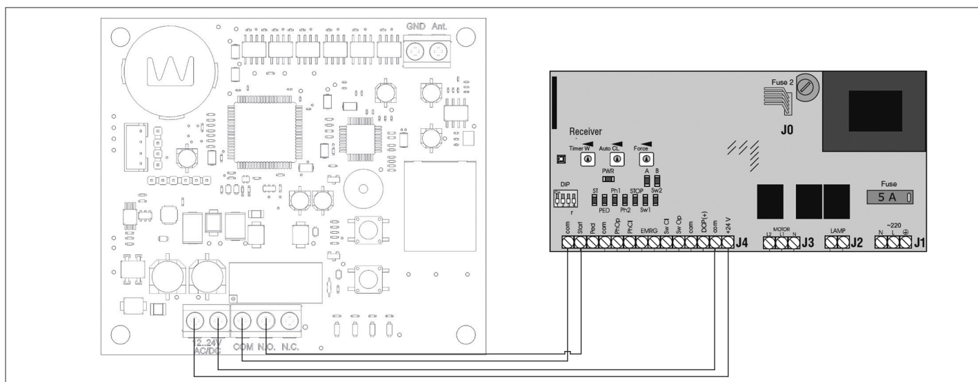
Рис. 1. Схема подключения Radioparking к плате PCB-SL
